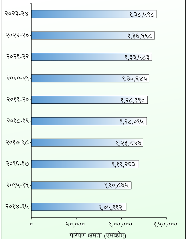
आलेख ९.७ : महापारेषणची वीज पारेषण क्षमता
