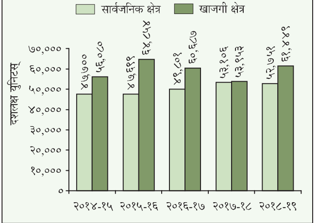
आलेख ९.२ : राज्यातील सार्वजनिक व खाजगी क्षेत्रातील वीज निर्मिती
